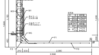
擁壁高さ:1,600mm 必要地耐力:50KN/m 2 断面図:ML1-500-07
