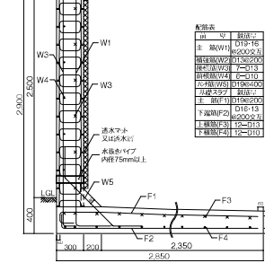
擁壁高さ:2,900mm 必要地耐力:100KN/m 2 断面図:L1-400-13
