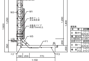
擁壁高さ:2,020mm 必要地耐力:95KN/m 2 断面図:ML1-350-09
