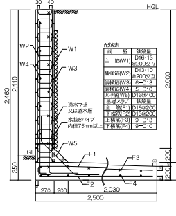
擁壁高さ:2,460mm 必要地耐力:85KN/m 2 断面図:L1-400-11
