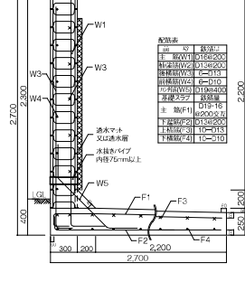
擁壁高さ:2,700mm 必要地耐力:95KN/m 2 断面図:L1-400-12
