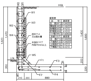
擁壁高さ:1,820mm 必要地耐力:90KN/m 2 断面図:ML1-350-08
