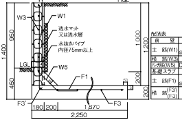
擁壁高さ:2,020mm 必要地耐力:60KN/m 2 断面図:L1-500-09
