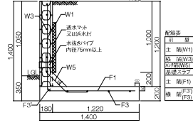
擁壁高さ:2,020mm 必要地耐力:75KN/m 2 断面図:L1-400-09
