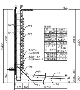
擁壁高さ:2,460mm 必要地耐力:70KN/m 2 断面図:L1-500-11
