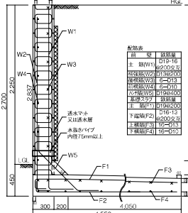
擁壁高さ:2,700mm 必要地耐力:75KN/m 2 断面図:L1-500-12
