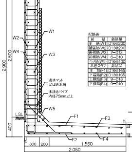
擁壁高さ:2,900mm 必要地耐力:125KN/m 2 断面図:L1-350-13
