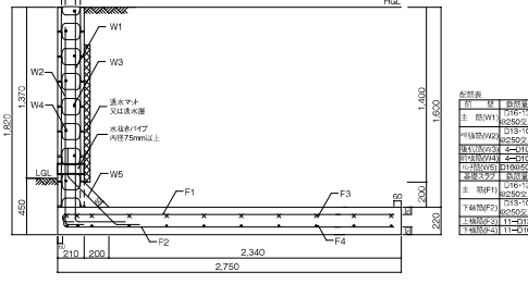
擁壁高さ:1,820mm 必要地耐力:55KN/m 2 断面図:ML1-500-08
