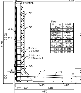
擁壁高さ:2,700mm 必要地耐力:120KN/m 2 断面図:L1-350-12
