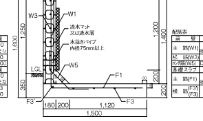
擁壁高さ:2,260mm 必要地耐力:80KN/m 2 断面図:L1-400-10
