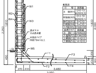
擁壁高さ:2,260mm 必要地耐力:65KN/m 2 断面図:L1-500-10
