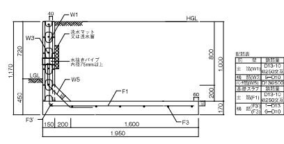
擁壁高さ:1,170mm 必要地耐力:40KN/m 2 断面図:ML1-500-05
