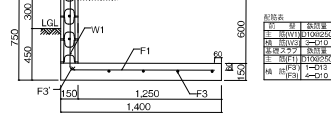
擁壁高さ:1,170mm 必要地耐力:40KN/m 2 断面図:ML1-500-05
