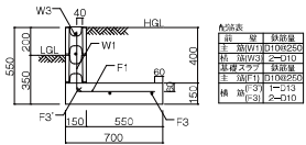
擁壁高さ:950mm 必要地耐力:45KN/m 2 断面図:ML1-400-04
