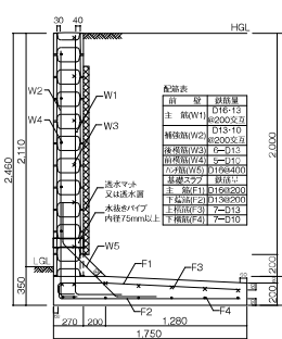
擁壁高さ:2,460mm 必要地耐力:110KN/m 2 断面図:L1-350-11
