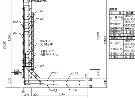
擁壁高さ:2,020mm 必要地耐力:95KN/m 2 断面図:ML1-350-09
