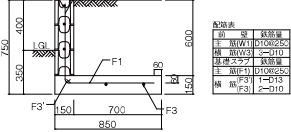
擁壁高さ:1,170mm 必要地耐力:55KN/m 2 断面図:ML1-400-05
