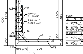
擁壁高さ:2,260mm 必要地耐力:100KN/m 2 断面図:L1-350-10
