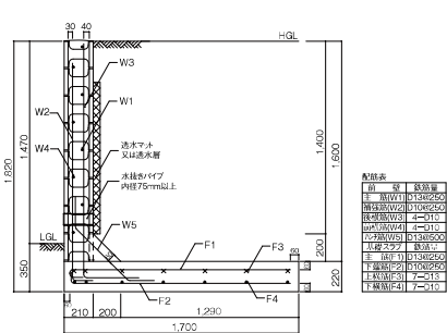
擁壁高さ:1,820mm 必要地耐力:75KN/m 2 断面図:ML1-400-08
