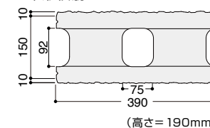
基本形横筋
