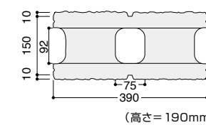
基本形横筋
