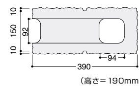
コーナー
