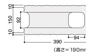
コーナー
